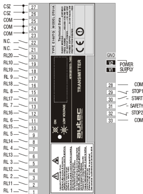
Sendereinheit
